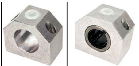
SA : palier seul
