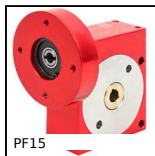
PF15 Réducteur à roue et vis sans fin, jusqu'à 3,75 Nm
