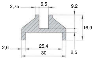
Profil type PGT-S
