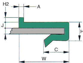
PRZ-C profil à clipser
