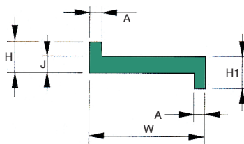
PRZ-P profil à poser
