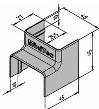
Angle PRF45-GOU-A
