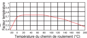
Fig.1-Facteur température (Ft)
