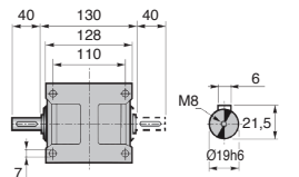
Arbre sortie simple S ou double B
