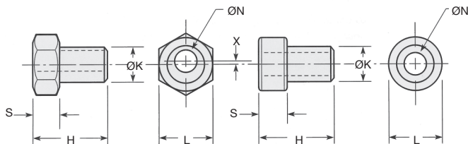
Douille excentrique réglable HBM-X
