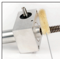
Dépolissage de zone difficilement accessible
