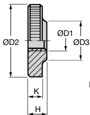
DIN 467
