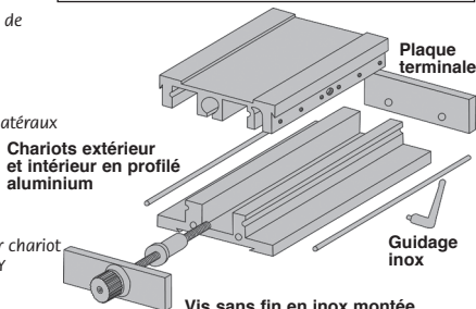
Vis sans fin en inox montée sur billes dans la plaque terminale
