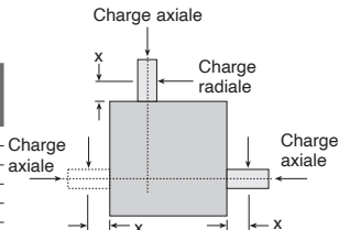
Renvoi d'angle BLHT
