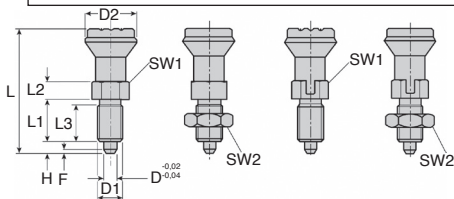
FORME A Sans contre-écrou Sans blocage FORME B Avec contre-écrou Sans blocage FORME C Sans contre-écrou Avec blocage FORME D Avec contre-écrou Avec blocage
