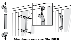
Montage sur profilé PRF
