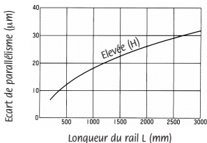
Fig.1 Parallélisme en fonctionnement
