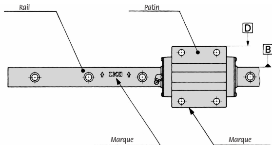
Fig.2 Surfaces de référence de montage
