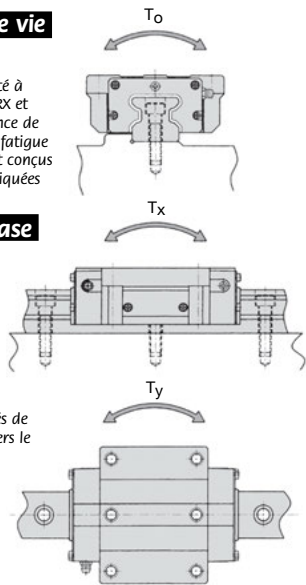
Figure 3 : Moment statique
