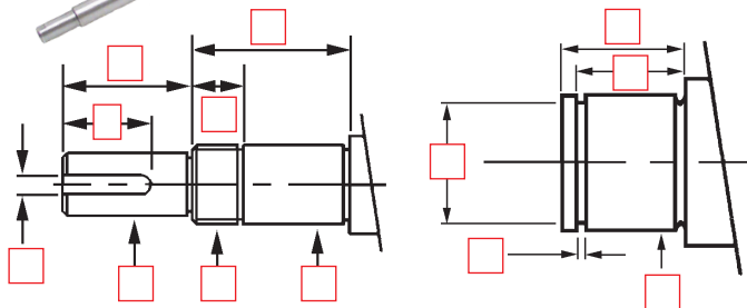
EXEMPLES D'EMBOUT
