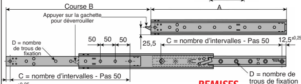
Plan : glissière gauche
