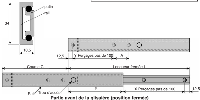
Partie avant de la glissière (position fermée)
