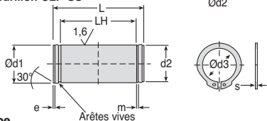
Tourillon CLP-SS
