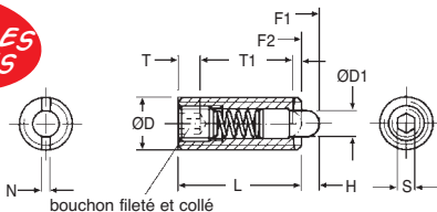
Corps acier doigt plastique
